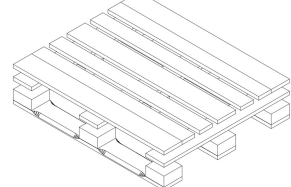
MESA DE ARMADO NAILING DESK
